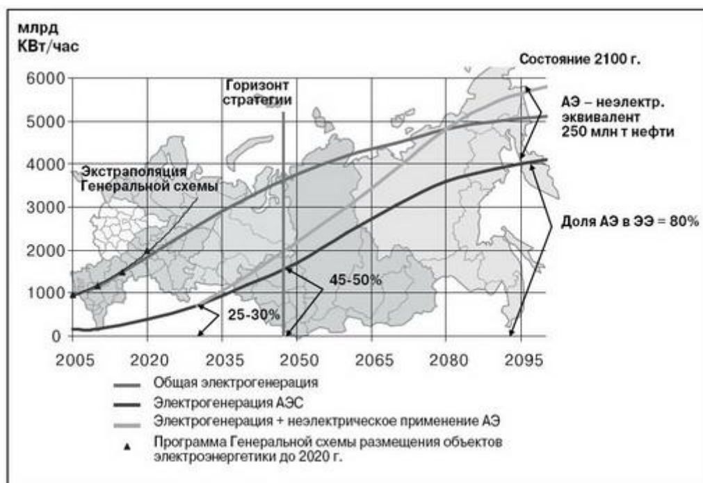
График 2. Развитие электроэнергетики (ЭЭ) России до 2100 г. и роль атомной энергетики (АЭ)
