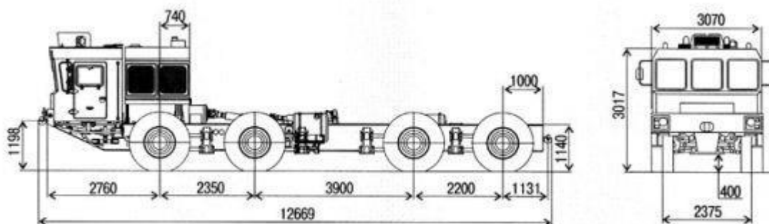
Рис. 2. Схема шасси МЗКТ-7930. Источник: Volatdefence.com
