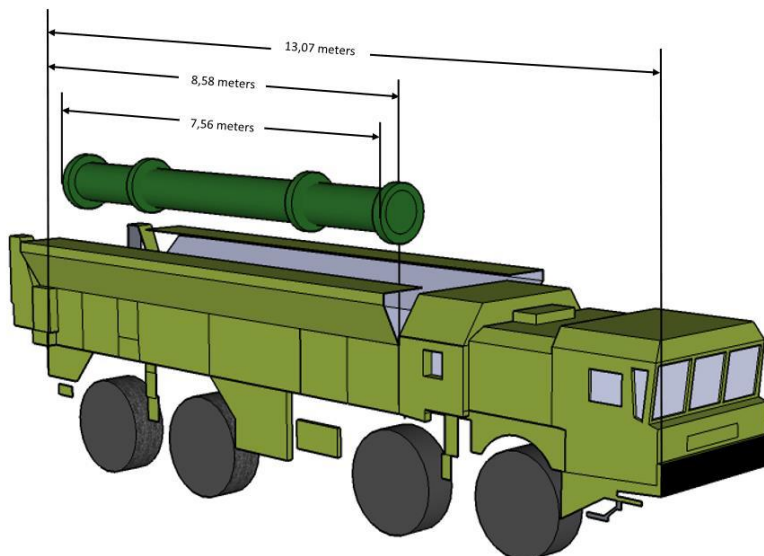
Рис. 3. Модель, полученная автором в Google SketchUp
